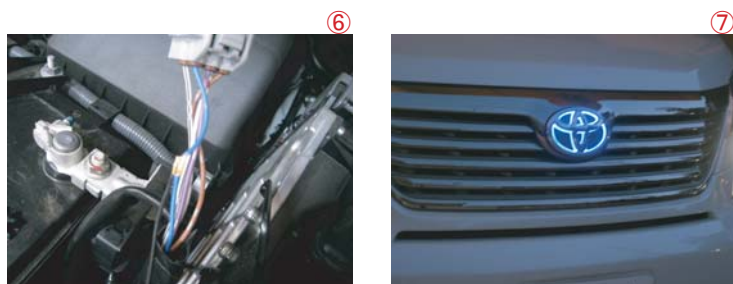
⑥ 配線はヘッドライトメインハーネスから+電源をとります。弊社確認時は青色がポジションランプ+線と確認しております。-線はボディアースに接続します。 ⑦ 配線の干渉等を確認後、取り外したパーツを元通りに組み上げて終了です。
